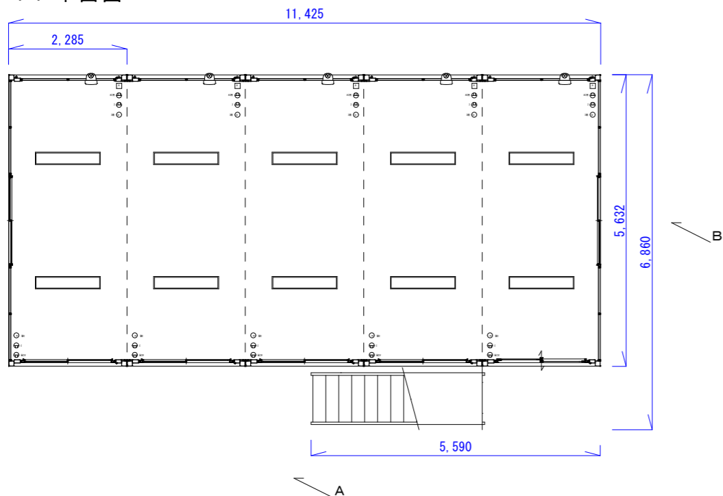
1 F 平面図
