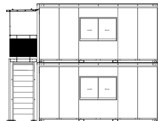
B 立面図
