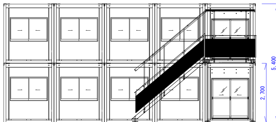
A 立面図
