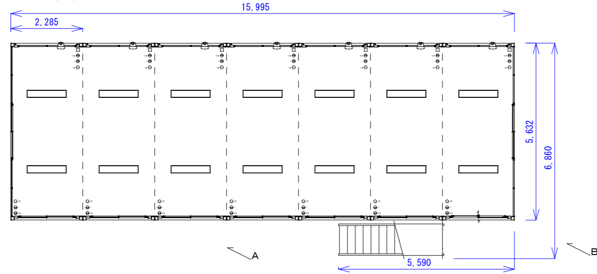
1 F 平面図
