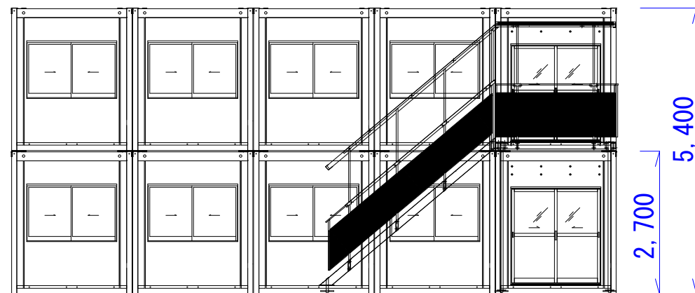
A 立面図
