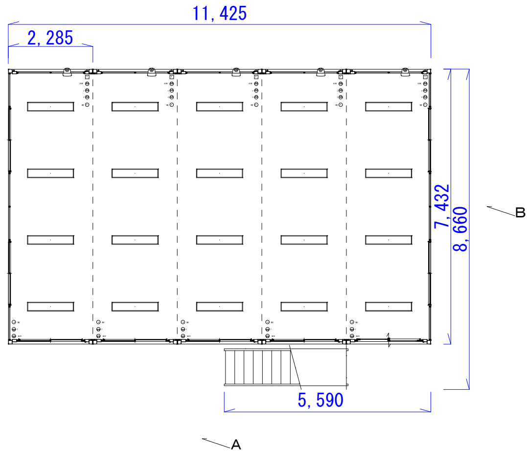
1 F 平面図
