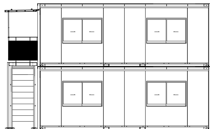
B 立面図
