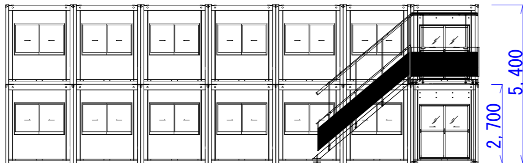
A 立面図
