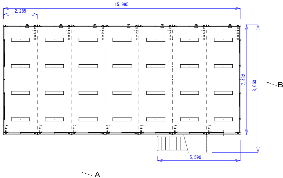
1 F 平面図
