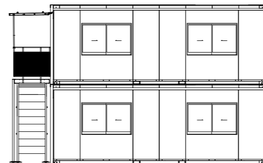
B 立面図
